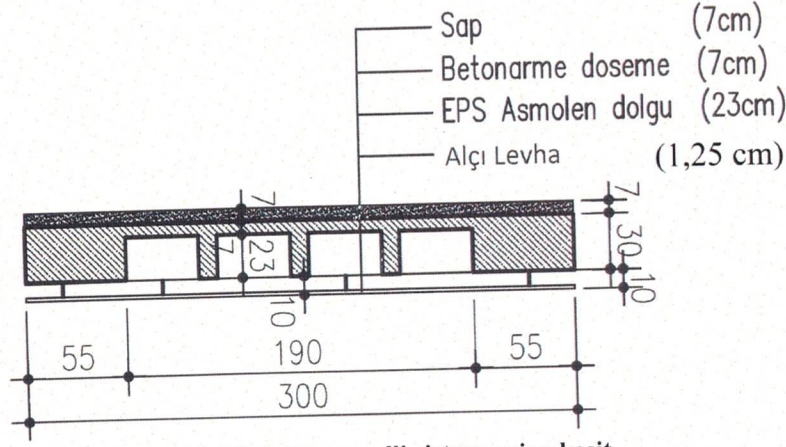
Şekil-4 Alçı panelli sistem enine kesit
